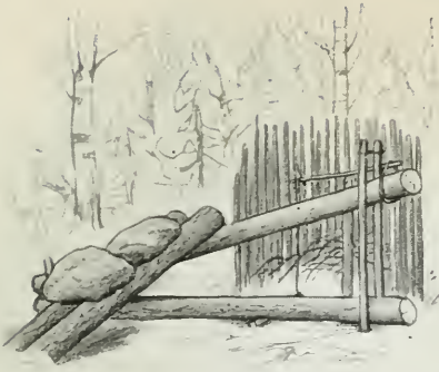
24. Jäniksen kahaloukku.
