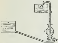
Montgolfier'n vesipuskuri.
