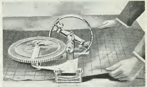
Mittakone.
