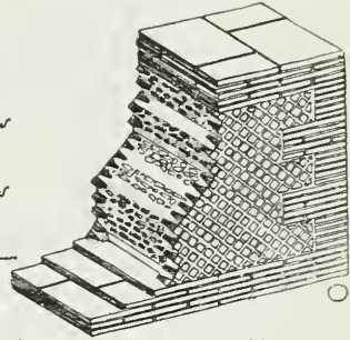
5. Roomalaista n. s. verkkomuuria (opus reticulatum).
