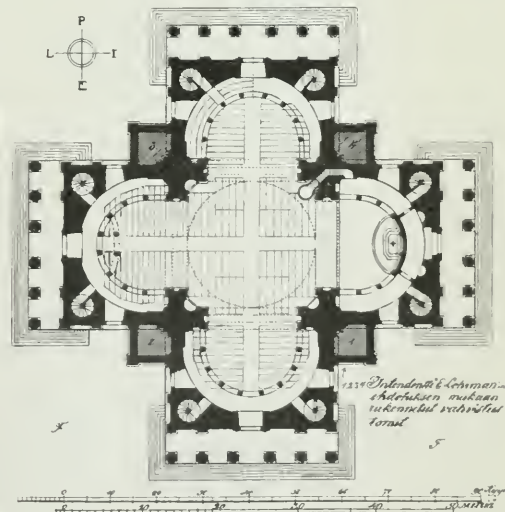
Kirkon pohjapiirustus.
