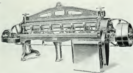
Halkaisukone.
