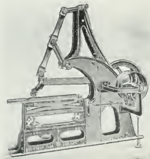
Kiillotuskone.
