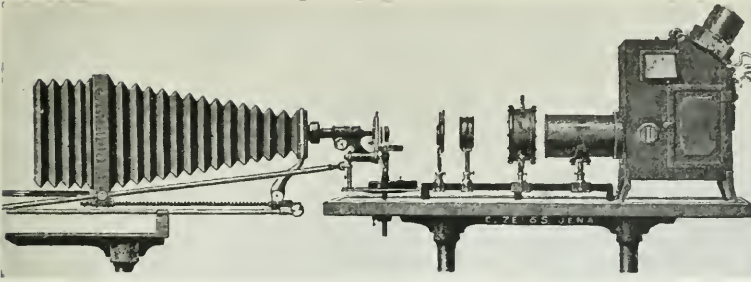
Vaakasuurassa asennossa oleva Zeissin mikrovalokuvauskone.
