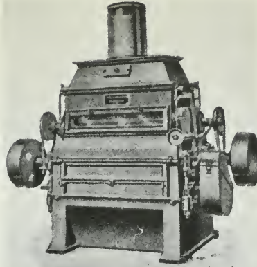
Kuva 2. Valssimylly.
