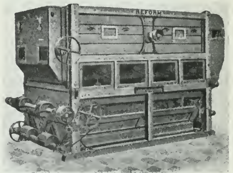
Kuva 6. Reform niminen puhdistuskone.
