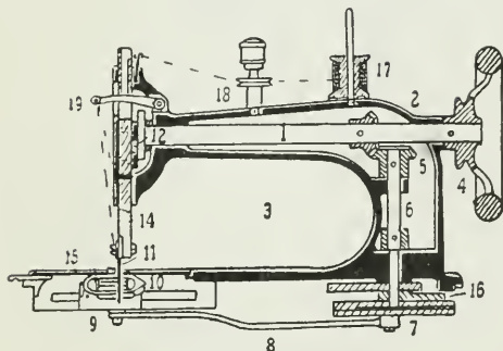
Singerkoneen leikkaus.
