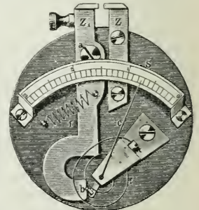
Mikrometri-avain.
