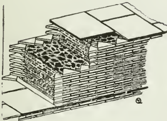
6. Roomalaista tiilillä päällystettyä täytemuuria.
